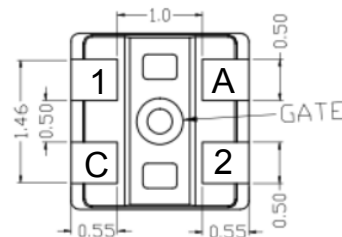
Bottom Side
